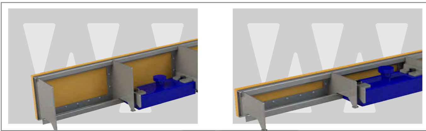
CLAMPING BRACKET FOR MF BASE PROFILE/ PINZAS SUJECIÓN IMÁN A ENCOFRADO MF/ PINCES DE FIXATION DES AIMANTS AU COFFRAGE/ ЗАЖИМЫ ДЛЯ ОПАЛУБКИ MF
